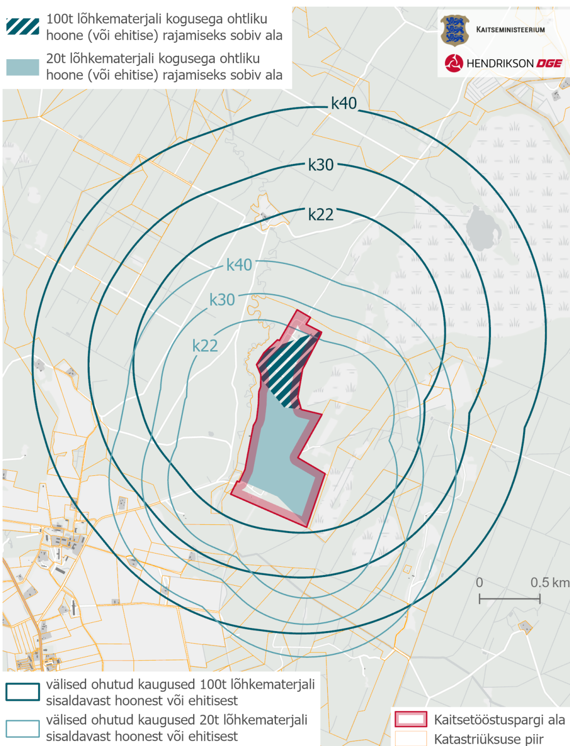
Joonis 2. Piirsalu ala välised ohutud kaugused. Lõhkematerjalide kogused on esitatud TNT ekvivalentides.
